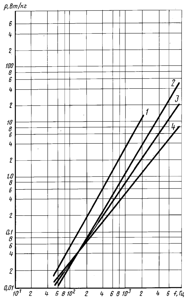
Зависимость P_{0.5} от частоты для сплавов марок: 1 — 81НМА толщиной 0,2 мм; 2 — 81НМА и 83НФ толщиной 0,1 мм; 3 — 81НМА и 83НФ толщиной 0,05 мм; 4 — 83НФ толщиной 0,02 мм
