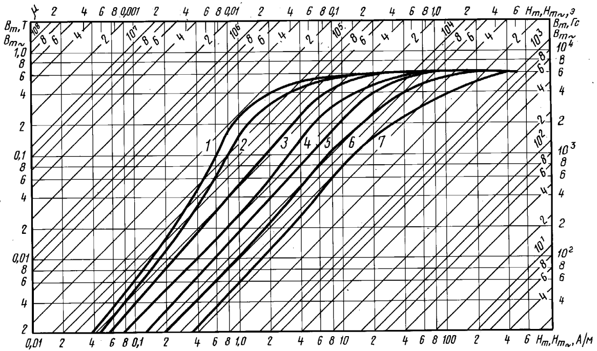
Кривые намагничивания сплава марки 80NХС толщиной 0,2 мм для частот: 1 — 0 Гц; 2 — 50 Гц; 3 — 400 Гц; 4 — 1000 Гц; 5 — 2000 Гц; 6 — 4000 Гц; 7 — 10000 Гц
