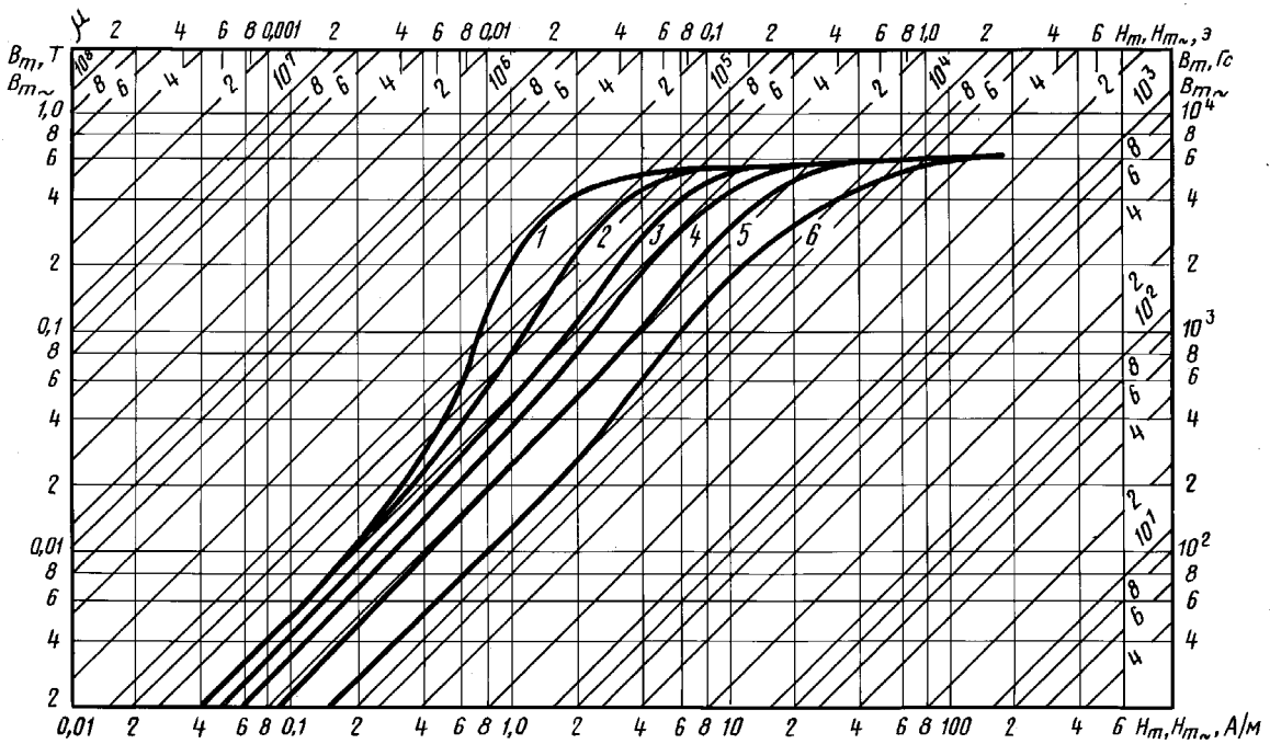
Кривые намагничивания сплава марки 80NХС толщиной 0,1 мм для частот: 1 — 0 Гц; 2 — 400 Гц; 3 — 1000 Гц; 4 — 2000 Гц; 5 — 4000 Гц; 6 — 10000 Гц
